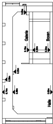
Schnitt
